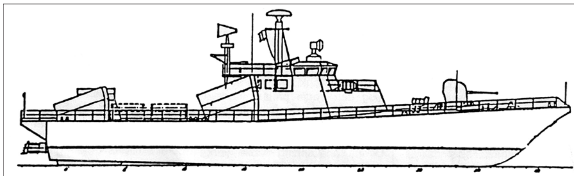
Ritning till en ny robotbåt av den s.k. Helsinki II-klassen. Displacement 200 ton, längd 40 m och bredd 7 m. Hastigheten överstiger 30 knop.
